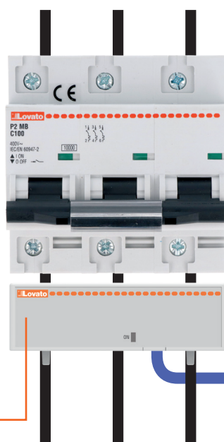
EXS3080 Трехфазный электронный трансформатор тока 80 А с кабелем RJ45 (2 м)
