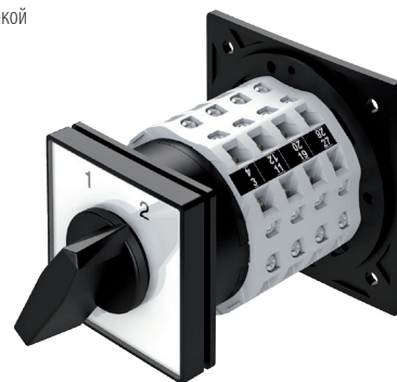
Установка на задней стенке электрического шкафа с черной ручкой
