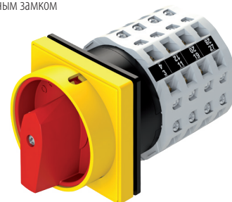
Фронтальная установка с красно-желтой ручкой, блокируемой навесным замком
